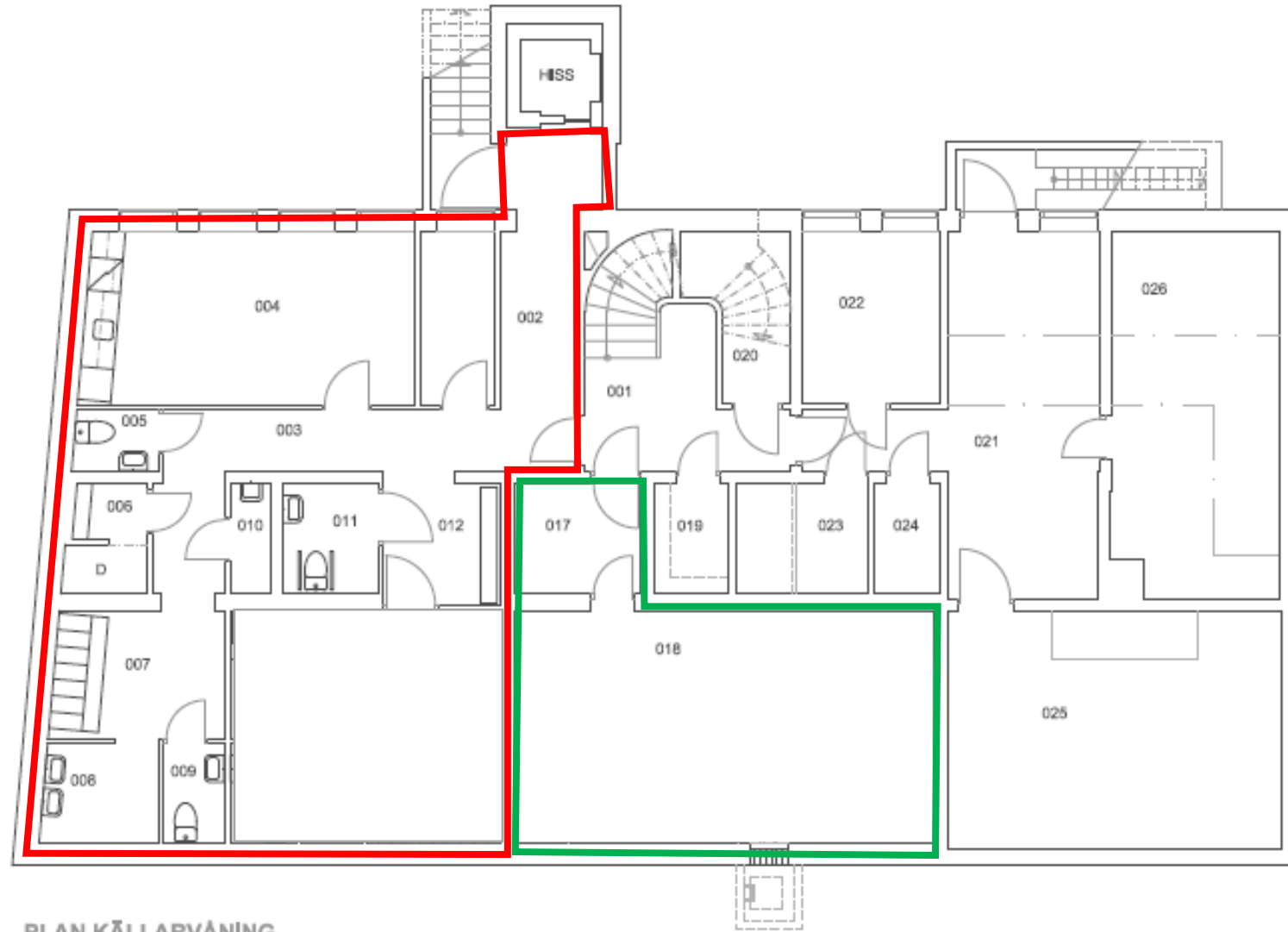
PLAN KÄLLARVÄNING
